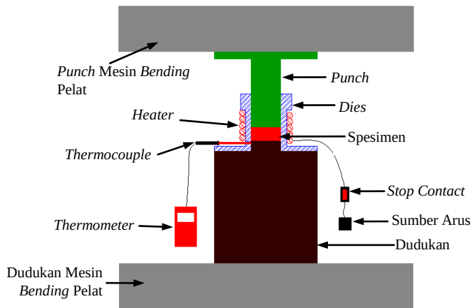
Gambar 5. Skema Proses Kompaksi
