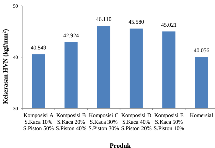
Gambar 9. Data Pengujian Kekerasan Terhadap Komposisi Produk Kanvas Rem
