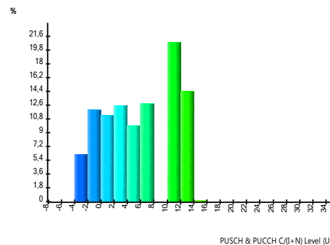
Gambar 4.6 Histogram cakupan CINR UL skenario 1
