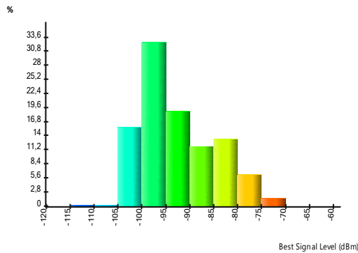
Gambar 4.2 Histogram Sinyal Level skenario 1
