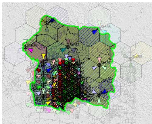
Gambar 3.9 Peletakkan eNodeB
