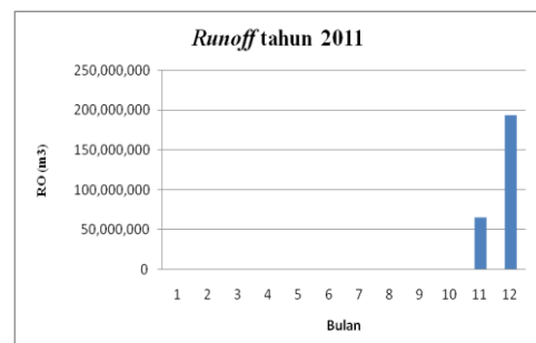
Gambar 7. Grafik Runoff tahun 2011
