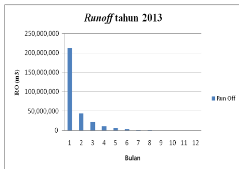
Gambar 9 Grafik Runoff tahun 2013
