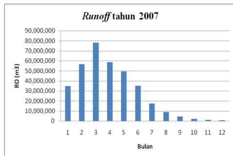
Gambar 3. Grafik Runoff tahun 2007
