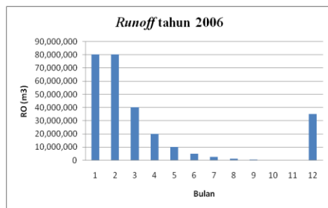
Gambar 2. Grafik Runoff tahun 2006
