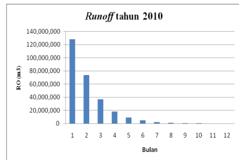
Gambar 6. Grafik Runoff tahun 2010
