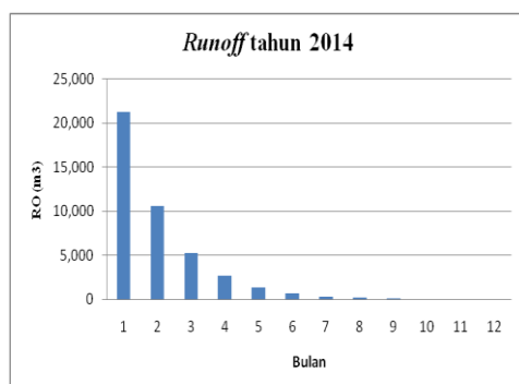
Gambar 10. Grafik Runoff tahun 2014
