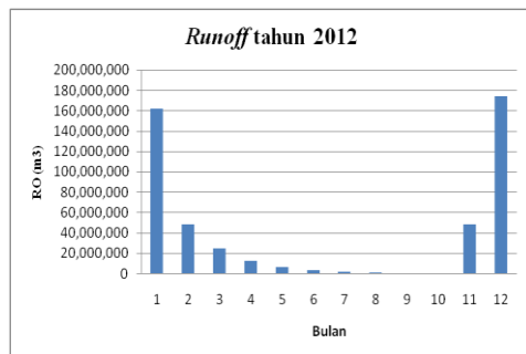
Gambar 8. Grafik Runoff tahun 2012
