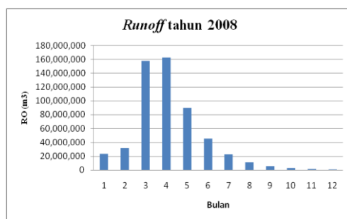
Gambar 4 Grafik Runoff tahun 2008
