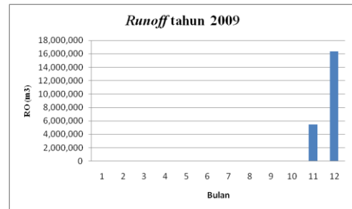
Gambar 5 Grafik Runoff tahun 2009
