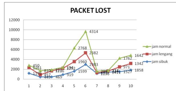
Gambar 8 Grafik Packet Lost Area Perkantoran
