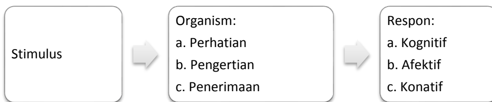
Gambar 1 Teori S-O-R
