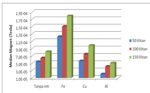
Gambar 4. Grafik pengaruh penambahan inti (Fe, Cu dan Al) terhadap medan magnetik pada coil dengan jumlah lilitan 50, 100 dan 150
