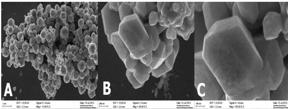
Gambar 5 : : Foto FESEM nanopartikel perak dengan konsentrasi larutan PVP 0.8 mmol dan volume larutan asam askorbit 0.20 mL. (A) Perbesaran 10.000 kali, (B) Perbesaran 50.000 kali, (C) Perbesaran 100.000 kali.
