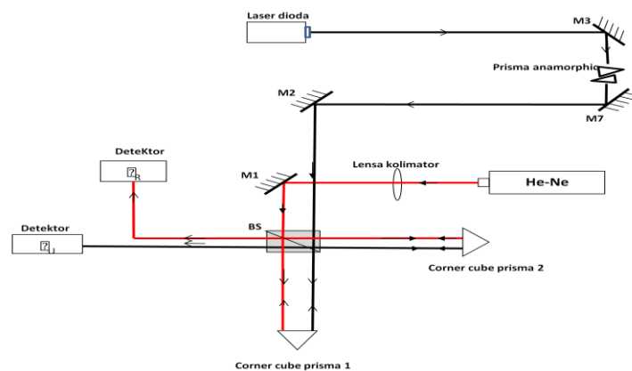
Gambar 1. Skema sistem rangkaian interferometer Michelson dengan dua sumber laser.
