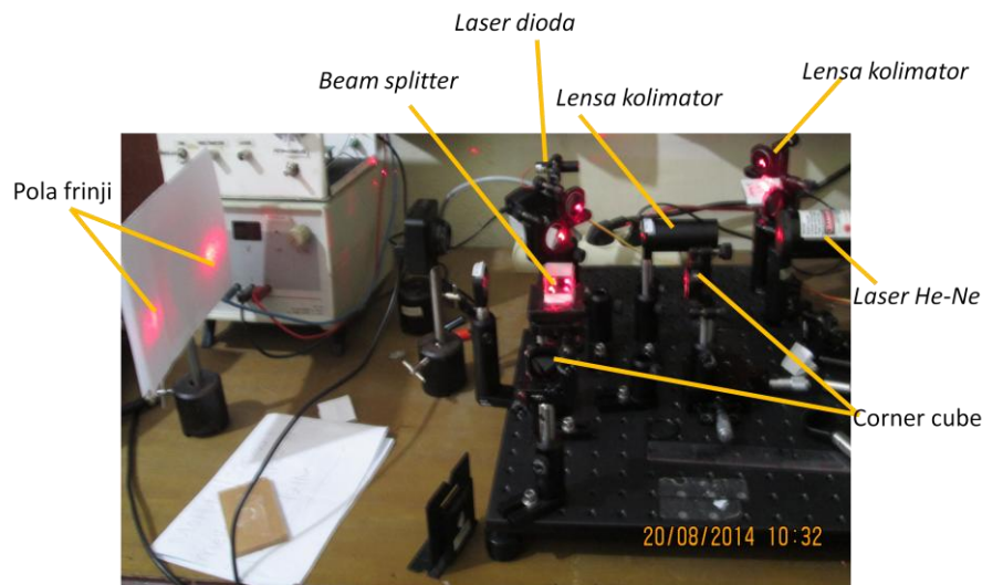
Gambar 2. Layout komponen optik dengan dua sumber laser
