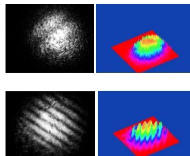
Gambar 3. Dua pola frinji yang berasal dari laser He-Ne (atas) dan laser dioda (bawah) pada sistem interferometer.
