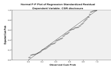
Gambar 1 Uji Normalitas
