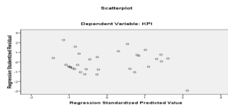
Gambar 2 Hasil Uji Heterokedastisitas
