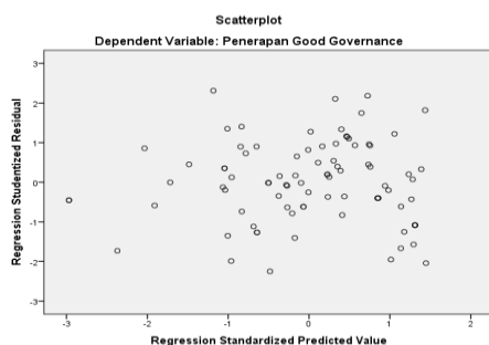
Gambar 1 Uji Heteroskedastisitas
