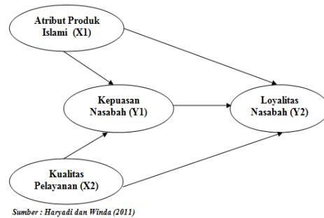
Gambar 1 Kerangka Penelitian
