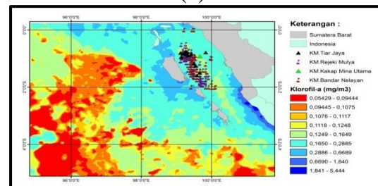
Gambar 2. Sebaran Konsentrasi Klorofil-a Musim Peralihan II Tahun 2013 (a) Bulan September (b) Bulan Oktober (c) Bulan November
