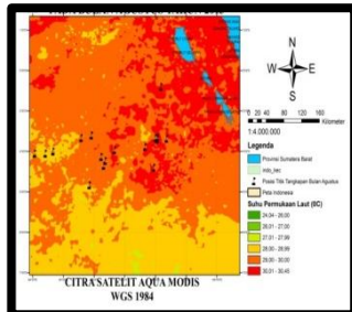
Gambar 13. Sebaran Suhu Permukaan Laut Musim Timur Bulan Agustus.
