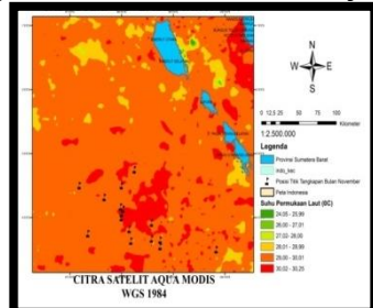
Gambar 16. Sebaran Suhu Permukaan Laut Musim Peralihan II
