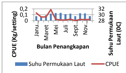
Gambar 18. Grafik CPUE Ikan Cakalang ( Katsuwonus pelamis )
