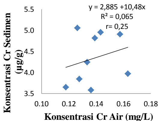
Gambar 5. Grafik Hubungan Konsentrasi Logam Cr pada Air Laut dengan Konsentrasi Cr pada Sedimen
