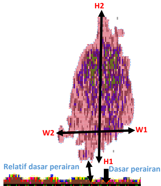
Gambar 6. Gambar Gerombol Memanjang Vertikal
