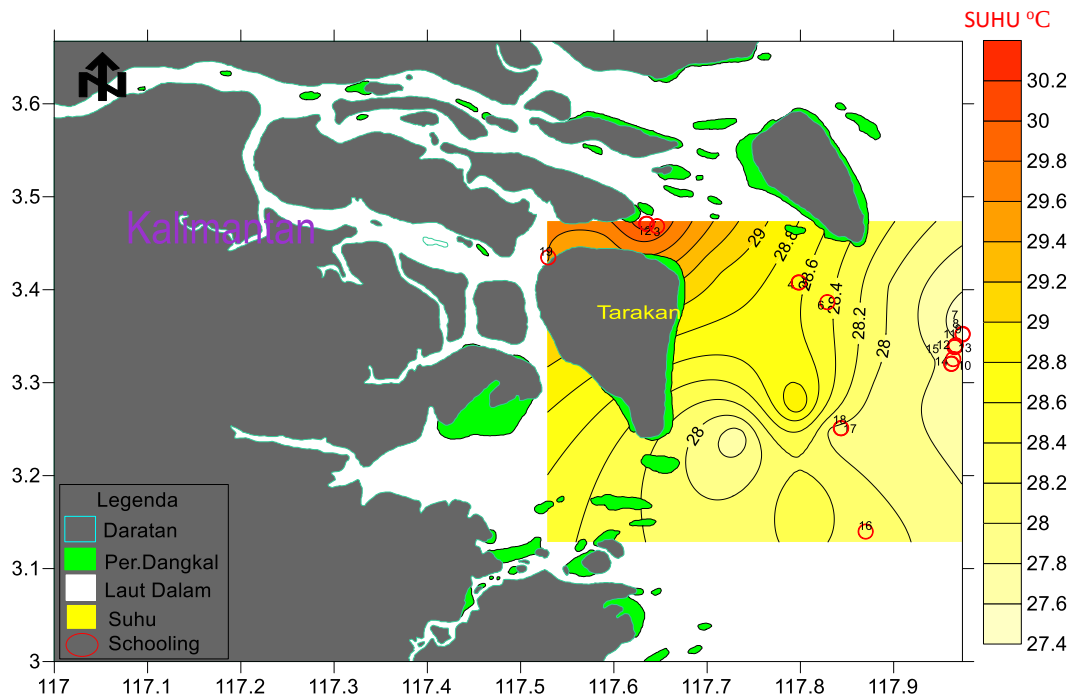
Gambar 4. Sebaran Suhu dan Gerombolan Ikan Di Perairan Tarakan
