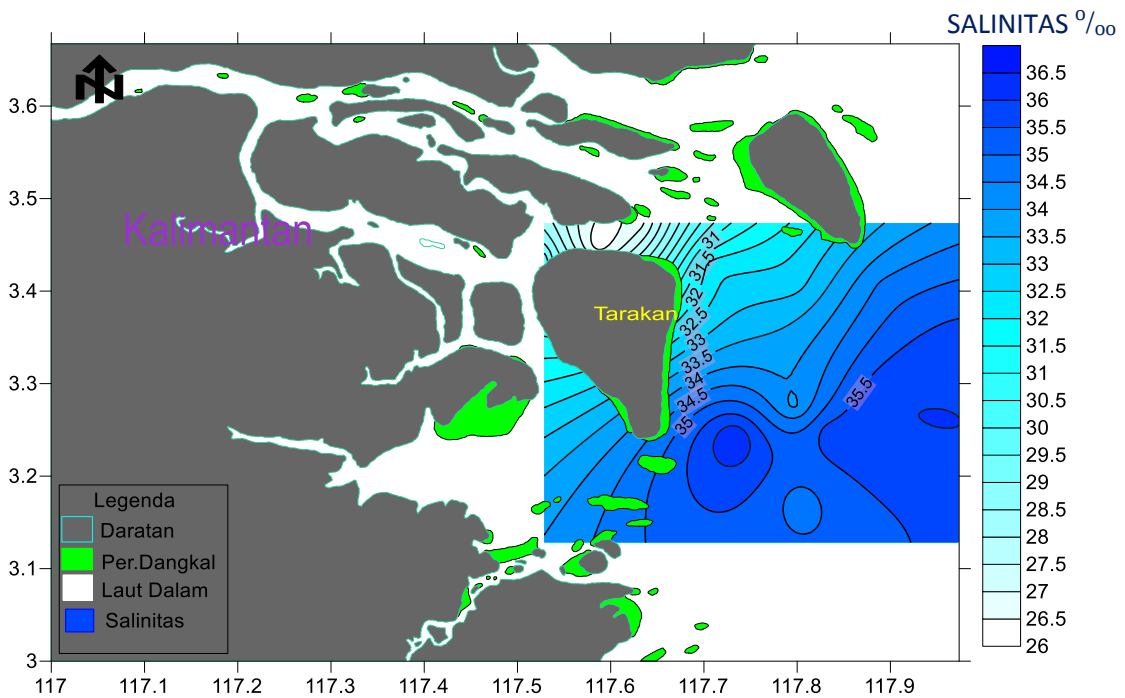
Gambar 3. Sebaran Salinitas di Perairan Tarakan
