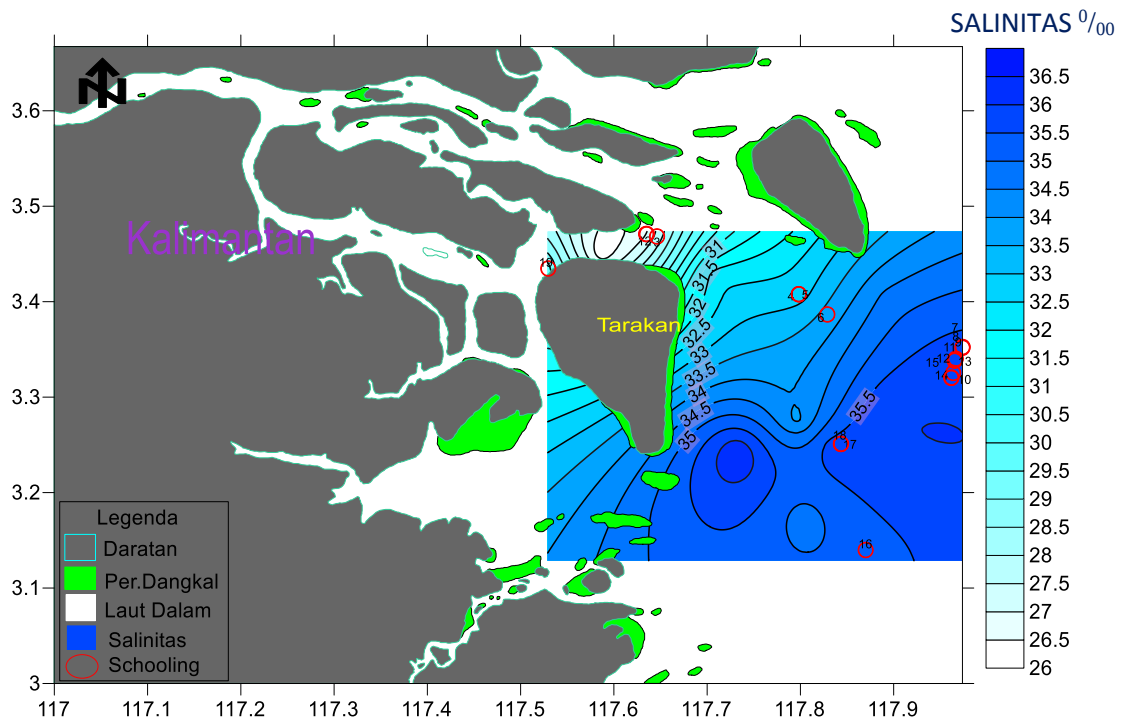
Gambar 5. Sebaran Salinitas dan Gerombolan Ikan Di Perairan Tarakan
