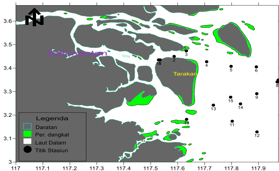
Gambar 1. Titik Stasiun Lokasi Penelitian di Perairan Tarakan
