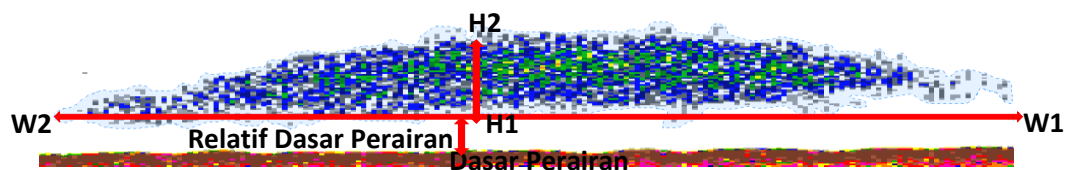
Gambar 7. Gerombolan Ikan Memanjang Horizontal
