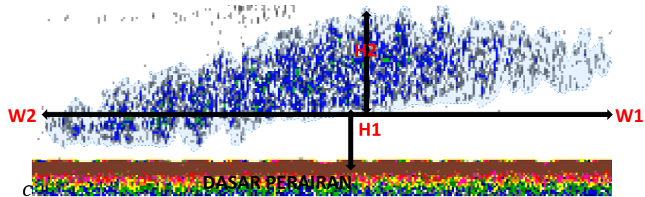
Gambar 8. Gerombol Ikan Memanjang Diagonal
