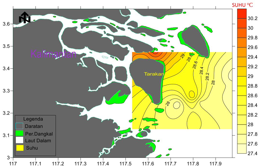
Gambar 2. Sebaran Suhu di Perairan Tarakan
